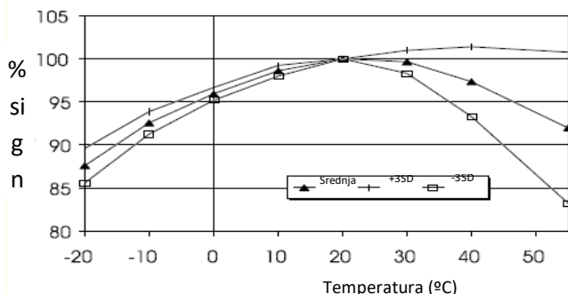
Zavisnost izlaznog signala od temperature
