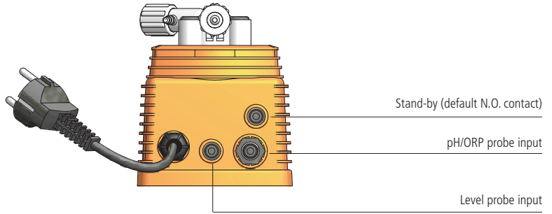
Fig. 10. Wirings
